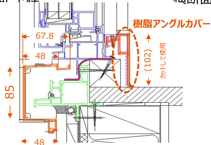
横断面 左縦枠
